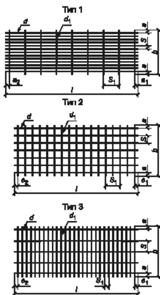
Рисунок 1 — Тяжелые сетки
