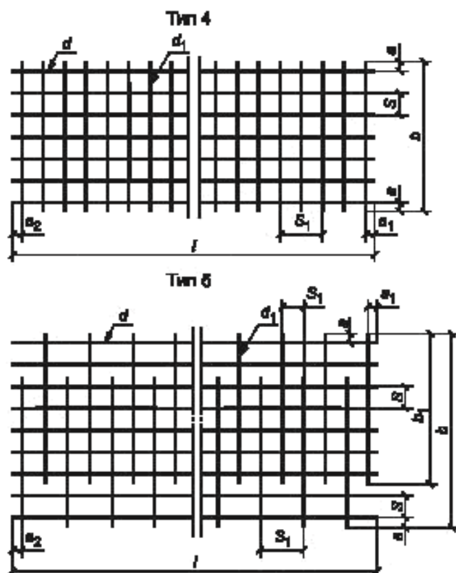
Рисунок 2 — Легкие сетки
